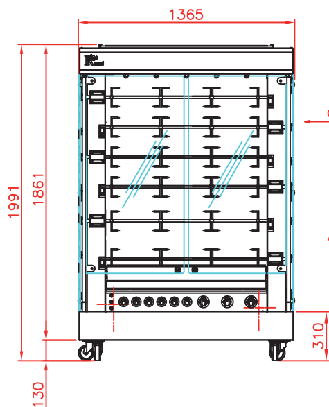
Vue de face Rôtissoire avec toit et socle à roulettes
