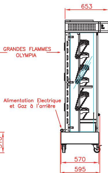
Vue de côté Rôtissoire avec toit et socle à roulettes
