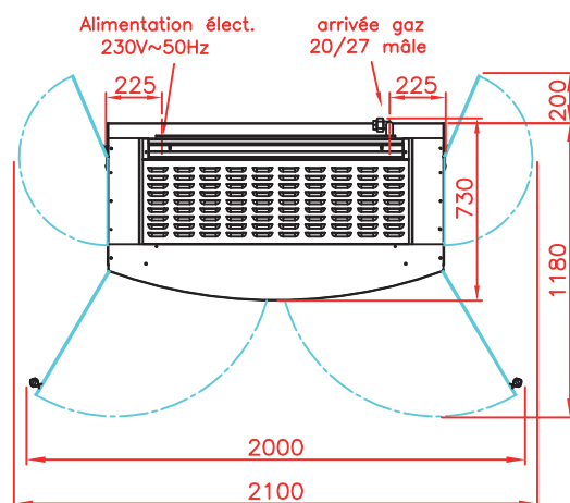
Vue de dessus Rôtissoire avec toit et socle à roulettes
