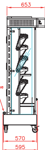
Vue de côté Rôtissoire avec toit et socle à roulettes
