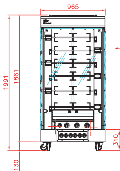
Vue de face Rôtissoire avec toit et socle à roulettes
